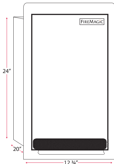
Fig. 1-1 Cutout dimensions
