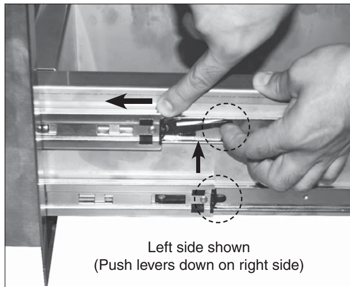
Fig. 1-2 Door removal
